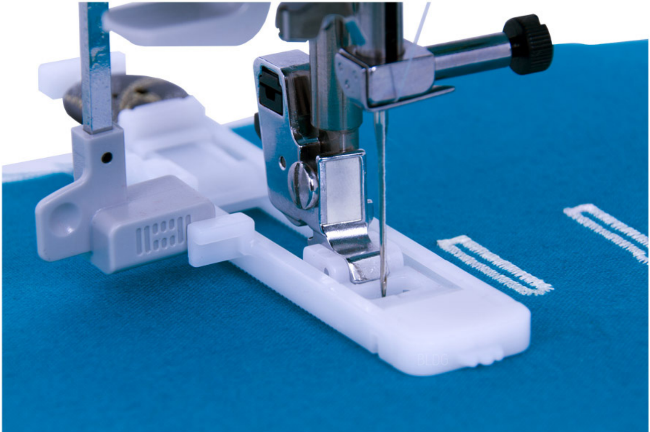
JUKI HZL-G100 Knopflochschiene
