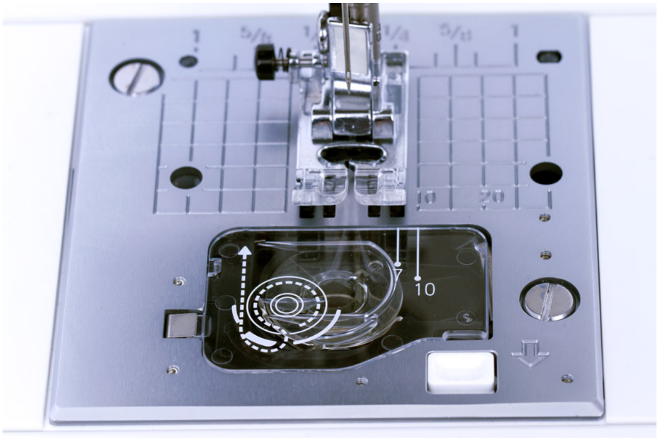
JUKI HZL-G100 Greifer
